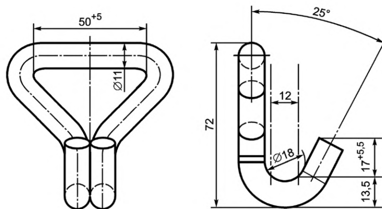
Рисунок 2 — Эталонный крюк
