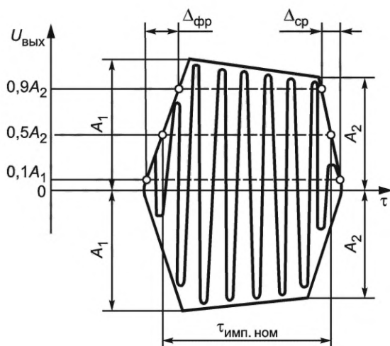
Рисунок 1 — Форма импульса
