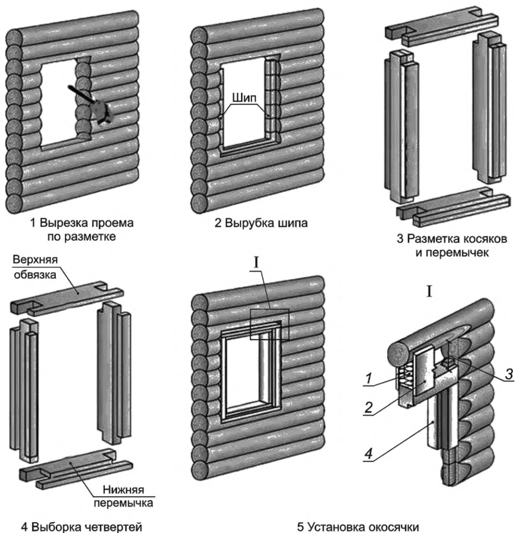
Рисунок Б.2 — Подготовка проема под установку короба (обсады)
