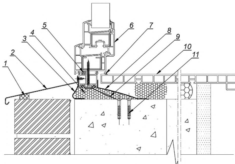
а) Узел нижнего примыкания в светопроемы зданий с двухслойной конструкцией стен
