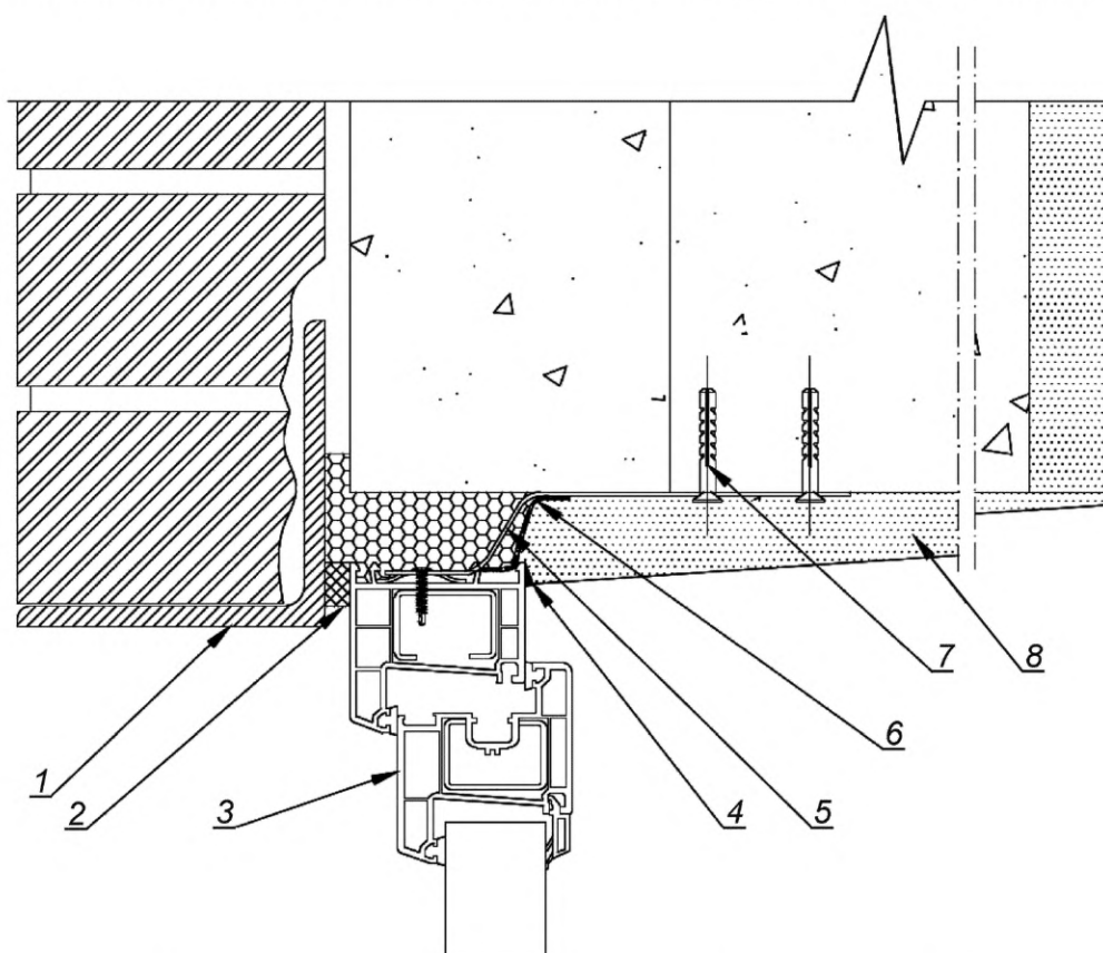
а) Узел нижнего примыкания в светопроемы зданий с двухслойной конструкцией стен
