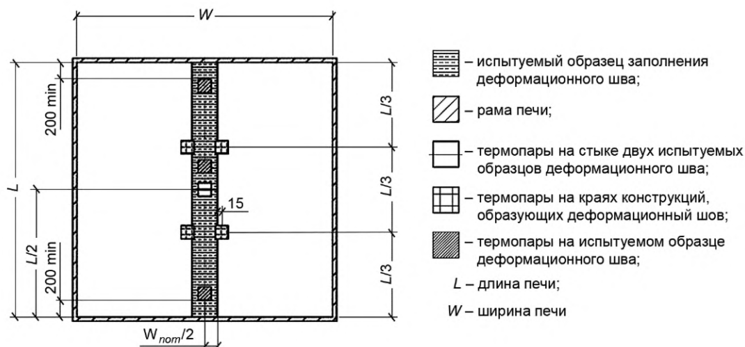
Рисунок 14 — Типовая схема расстановки термодатчиков (горизонтальная печь)
