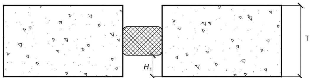
Рисунок 8 — Величина H_1
