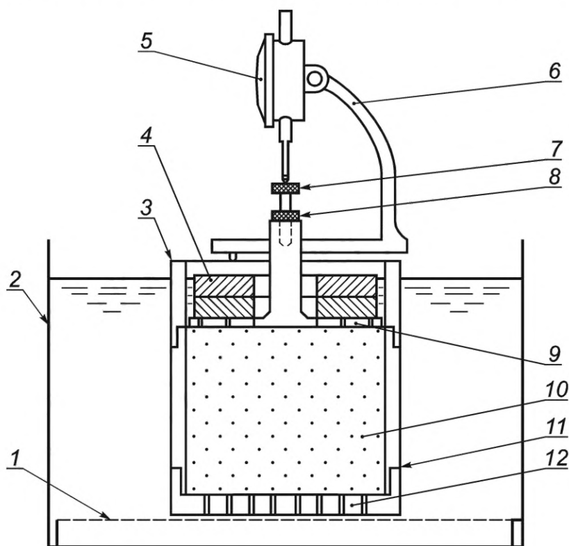
1 — подставка; 2 — емкость для воды; 3 — удлинительное кольцо; 4 — пригрузочный диск; 5 — индикатор часового типа; 6 — держатель индикатора часового типа; 7 — регулируемый стержень; 8 — контргайка; 9 — перфорированная пластинка; 10 — образец; 11 — цилиндрическая часть формы; 12 — перфорированное основание формы
