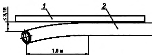
1 — поверочная линейка длиной не менее 1,6 м; 2 — труба
