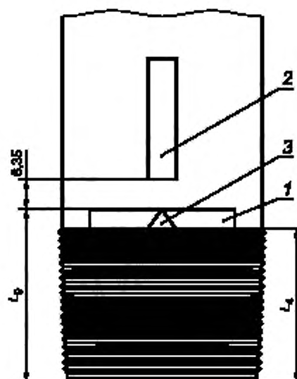
1 — полоса краской зеленого цвета; 2 — полоса краской на nipple'ном конце шириной приблизительно 25 мм и длиной приблизительно 0,6 м, если муфта будет установлена изготовителем длиной не менее 100 мм; 3 — треугольное клеймо; L_4 — общая длина резьбы от торца трубы до конца сбега резьбы; L_g — максимальная длина свинчивания: от торца трубы до вершины треугольного клейма
