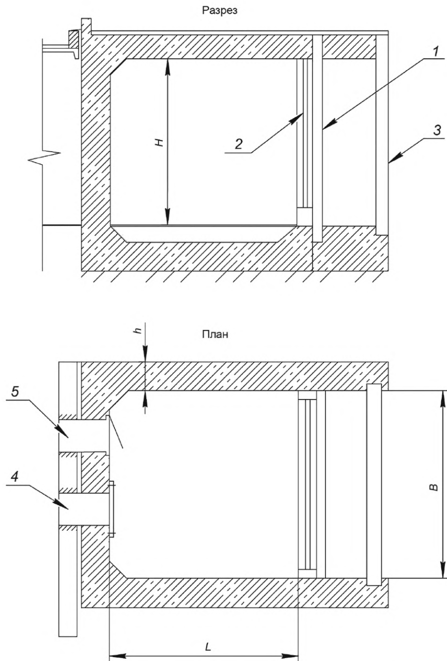
1 — перфоранель; 2 — легко разрушаемый утеплительный элемент; 3 — вышибная поверхность; 4 — проем; 5 — защитная дверь
