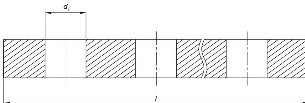
Рисунок 3 — Перфорированная панель
