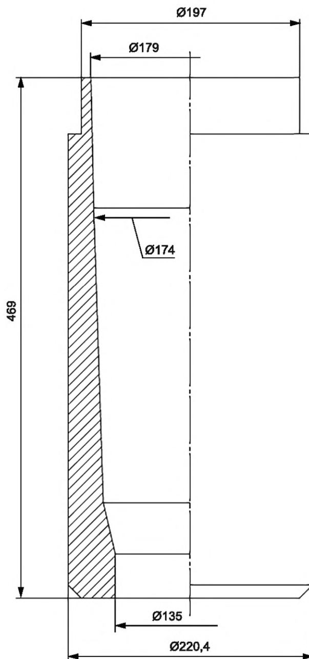
Рисунок 3 — Прошивная матрица
