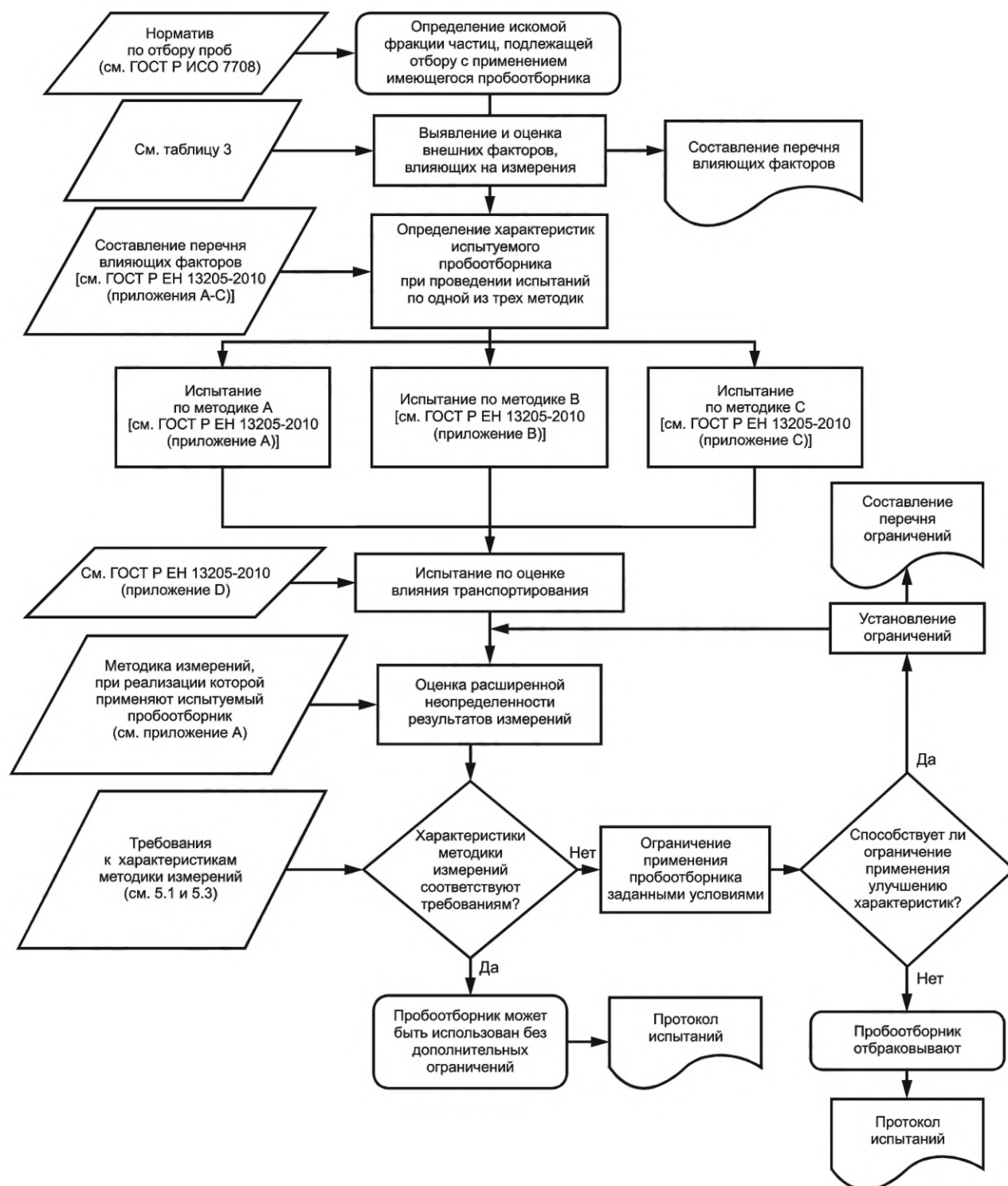
Рисунок 2 — Блок-схема для определения характеристик методики измерений, реализуемой с применением испытуемого пробоотборника (см. 7.2)
