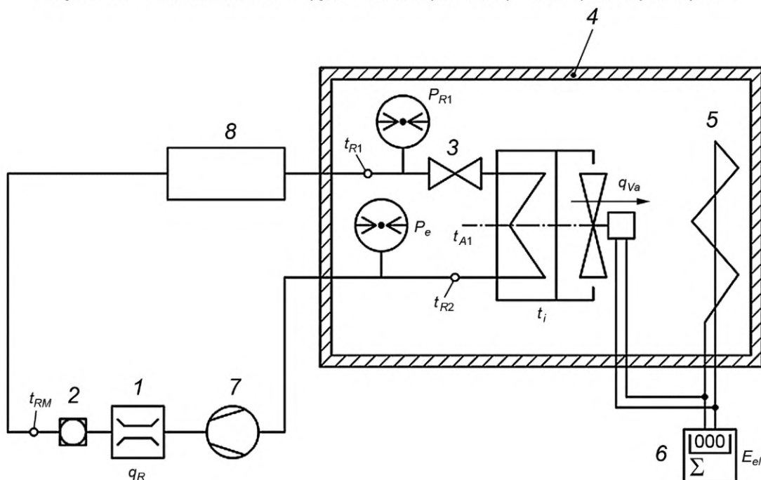
Рисунок Б.1 — Испытательное оборудование для работы в режиме прямого расширения
