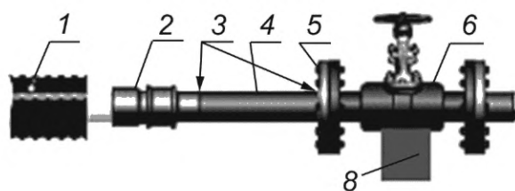
а) На фланцах
