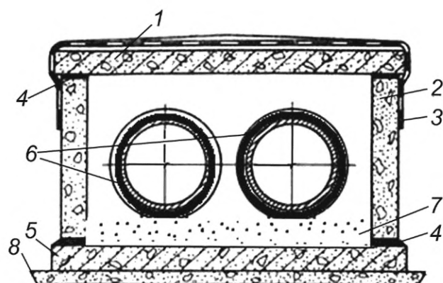
1 — плита перекрытия; 2 — стеновой блок; 3 — гидроизоляция; 4 — цементный раствор; 5 — плита днища; 6 — ТрК; 7 — просеянный песок; 8 — песчаная подготовка
