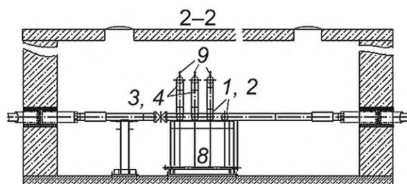
в) Вид 2-2
