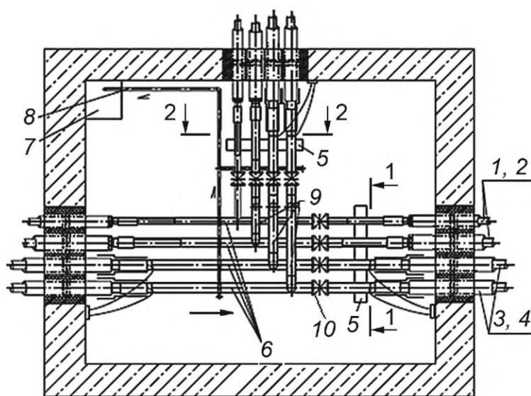
а) План
