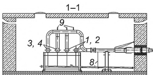
б) Вид 1-1
