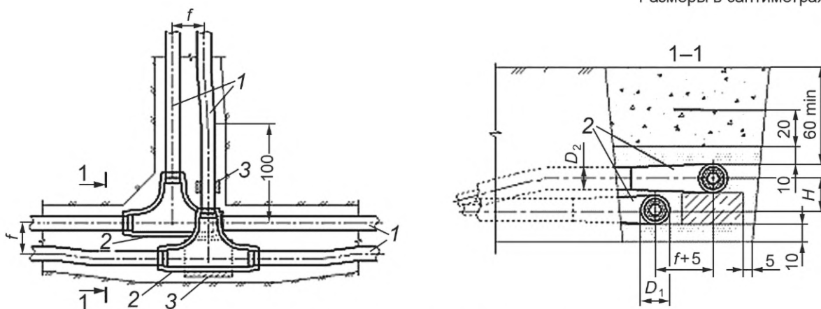
а) Прокладка ВГТгнт из двухтрубных ТрК
