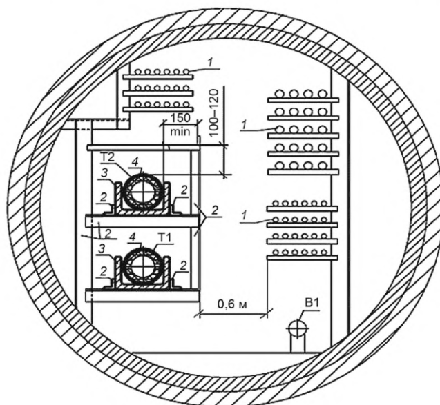
а) В тоннеле
