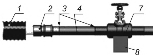
б) На сварке
