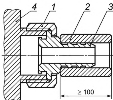
1, 3 — узел накидной гайки; 2 — стальная труба; 4 — жестко закрепленный штуцер
