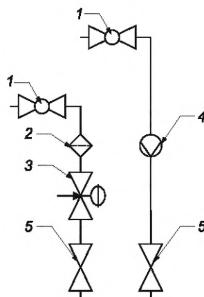
1 — запорная арматура с разъемными соединениями; 2 — сетчатый фильтр; 3 — автоматический комбинированный клапан — регулятор перепада с ограничением расхода; 4 — теплосчетчик; 5 — запорная арматура
