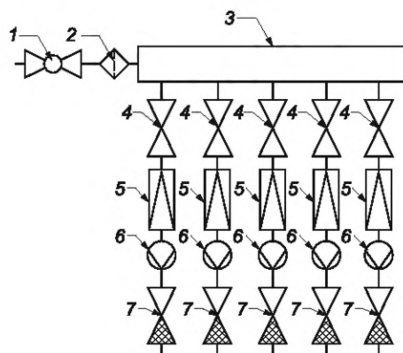
1 — запорная арматура с разъёмными соединениями; 2 — сетчатый фильтр; 3 — коллектор; 4 — запорная арматура; 5 — квартирный регулятор давления; 6 — водосчётчик; 7 — обратный клапан
