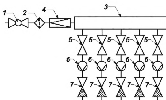
1 — запорная арматура с разъёмными соединениями; 2 — сетчатый фильтр; 3 — коллектор; 4 — квартирный регулятор давления; 5 — запорная арматура; 6 — водосчётчик; 7 — обратный клапан
