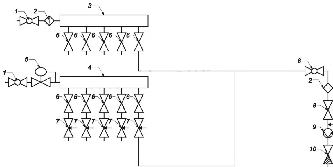
1 — запорная арматура с разъемным соединением; 2 — сетчатый фильтр; 3 — подающий коллектор; 4 — обратный коллектор; 5 — термостатический балансирующий клапан; 6 — запорная арматура; 7 — ручной балансирующий клапан; 8 — регулятор давления; 9 — водосчетчик; 10 — обратный клапан
