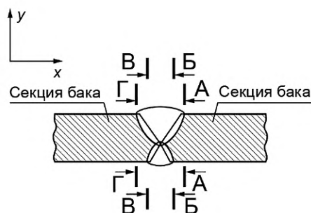
Рисунок Н.3 — Узел, образованный продольным стыковым сварным швом сварки секций бака (узел VI)
