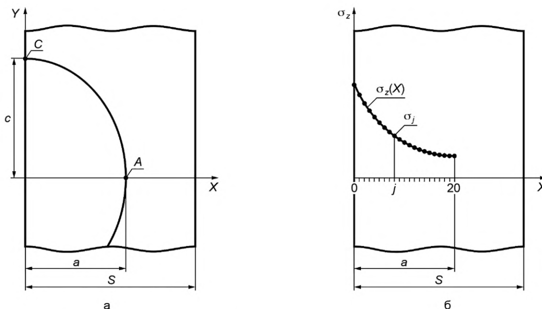
А, С — расчетные точки; а, с — малая и большая полуоси полуэллиптической трещины; S — толщина стенки компонента
