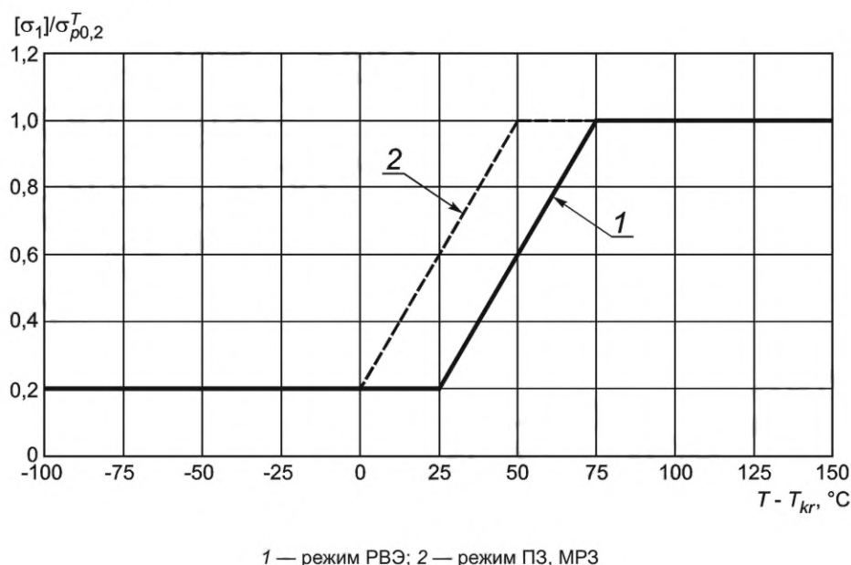
Рисунок 7.2 — Диаграмма допускаемых напряжений в элементах МК РБМК-1000 по критериям торможения разрушения
