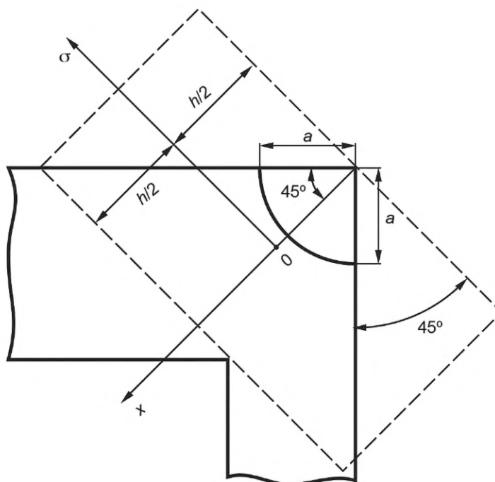
Рисунок М.3 — Четвертьэллиптическая поверхностная трещина в узле, образованном двумя пластинами, и схематизация расчетного параметра h
