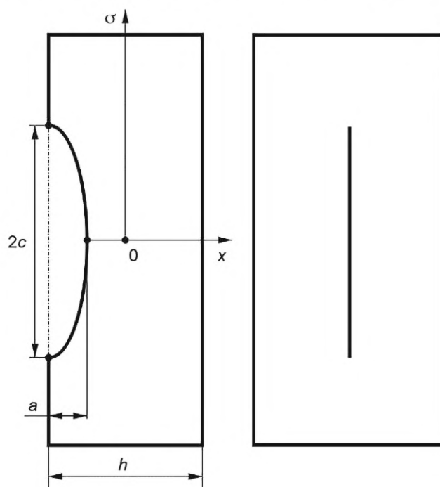
Рисунок М.1 — Полуэллиптическая поверхностная трещина в пластине
