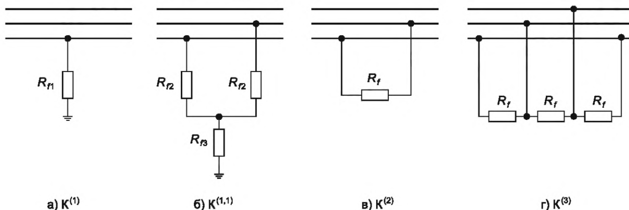
Рисунок А.1 — Схемы замещения КЗ
