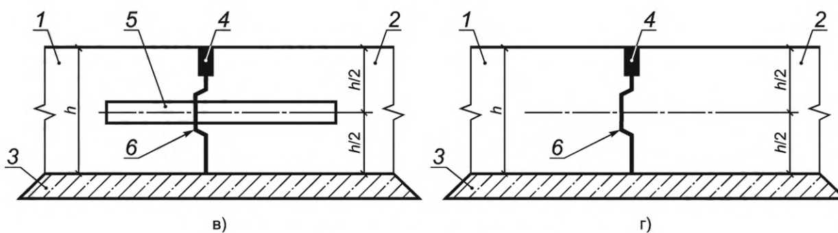
в), г) Шпунтовый тип трапецидального сечения
