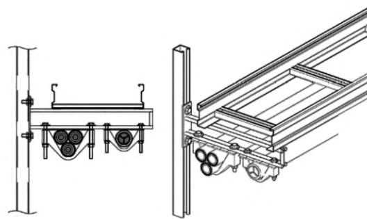
Рисунок Г.6 — Системы лестничных лотков или кабельроств, расположенные на верхнем ярусе двухуровневых полок и силовые кабели, расположенные на нижнем ярусе двухуровневых полок
