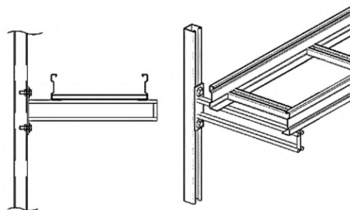
Рисунок Г.2 — Системы лестничных лотков или кабельроств, расположенные на верхнем ярусе двухуровневых полок
