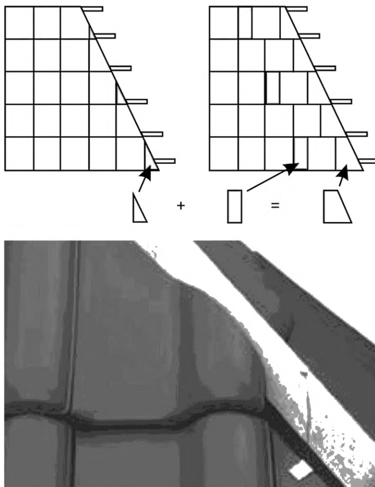
Рисунок 16 — Установка черепицы на хребте
