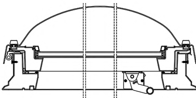
а — модуль с защитным куполом из монолитного поликарбоната и однокамерным стеклопакетом
