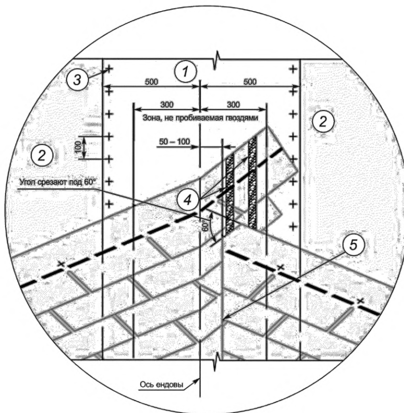
1 — подкладочный ковер; 2 — основание под черепицу (ОСП либо ФСФ); 3 — гвоздь; 4 — битумная мастика; 5 — линия подреза битумной черепицы
