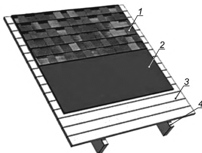
Рисунок 7 — Пример устройства сплошного основания из сплошного дощатого настила
