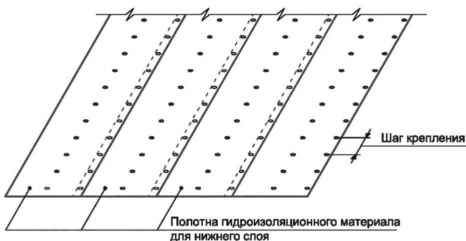
Рисунок 12 — Схема крепления материалов по центру рулона
