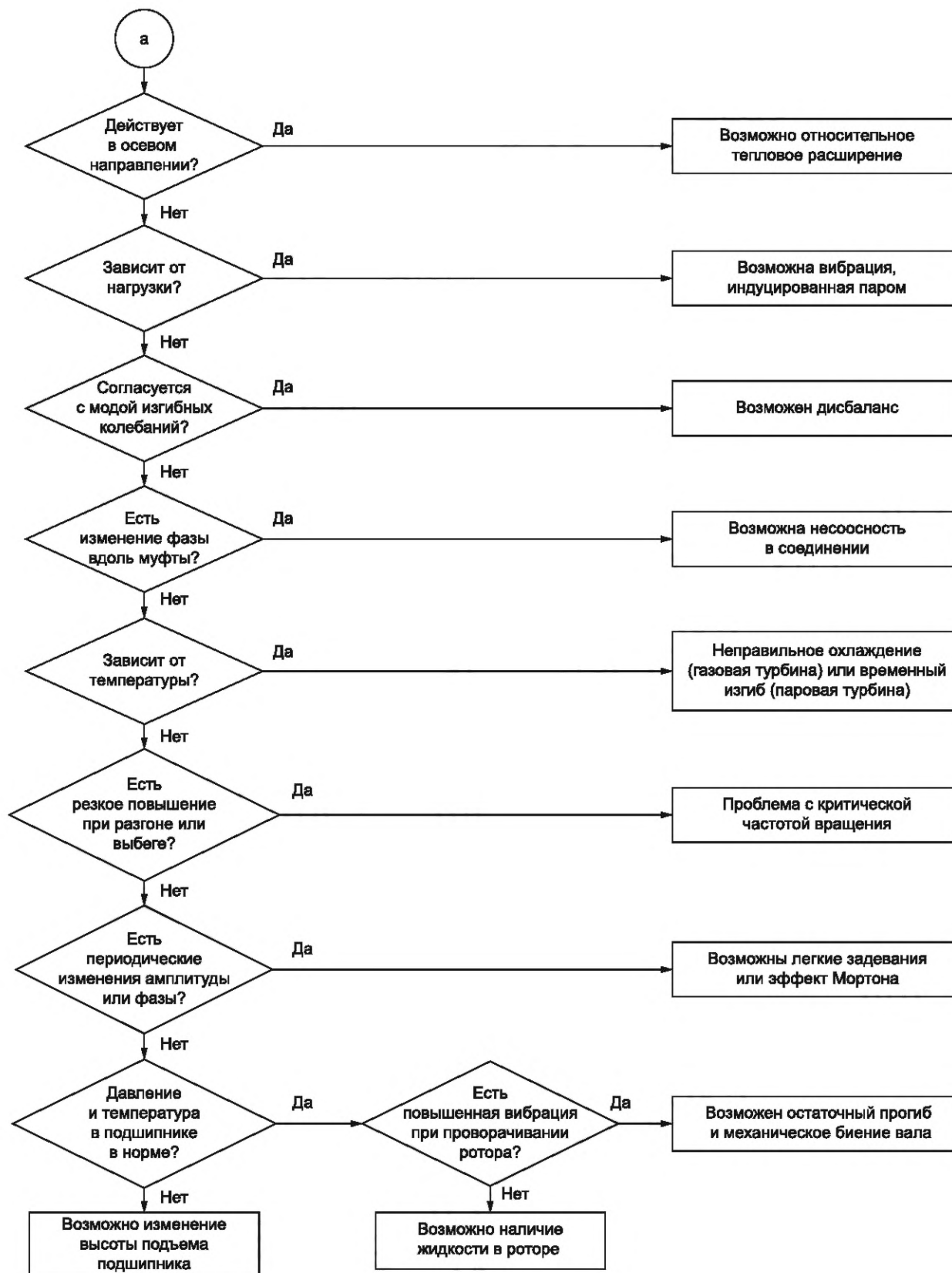
Рисунок В.2 — Схема диагностирования газовых и паровых турбин с гидравлическими подшипниками при повышенной вибрации на частоте вращения
