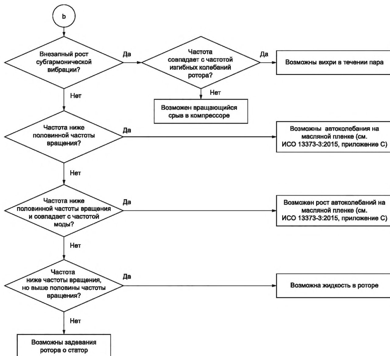
Рисунок В.3 — Схема диагностирования газовых и паровых турбин с гидравлическими подшипниками при наличии вибрации в области субгармонических частот
