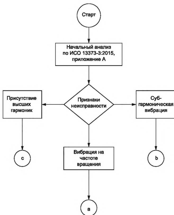
Рисунок В.1 — Схема вибрационного диагностирования газовых и паровых турбин с гидравлическими подшипниками
