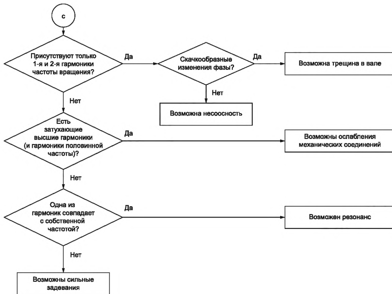
Рисунок В.4 — Схема диагностирования газовых и паровых турбин с гидравлическими подшипниками при повышенной вибрации на частоте вращения и ее гармониках
