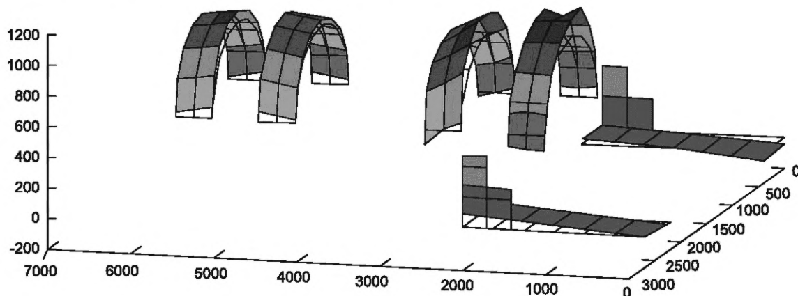
Рисунок С.5 — ODS на подшипниках турбины и опорной конструкции [12]
