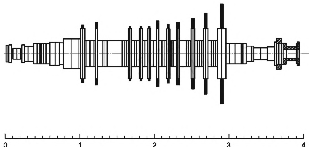
Рисунок С.3 — Схема турбины
