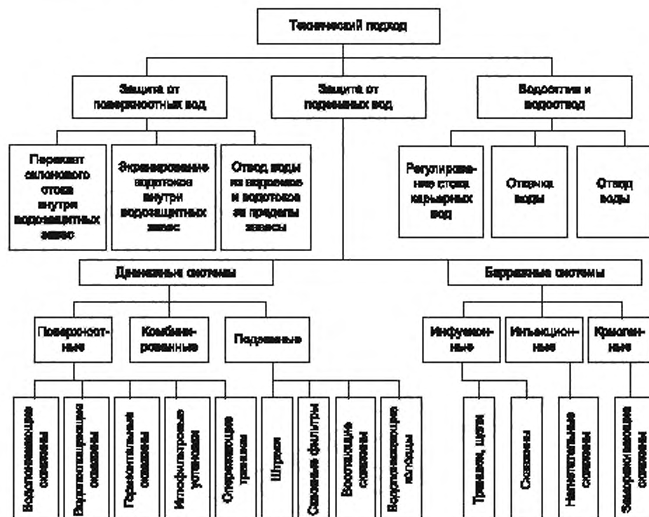
Рисунок В.1 — Мероприятия по снижению техногенного воздействия карьерных вод
