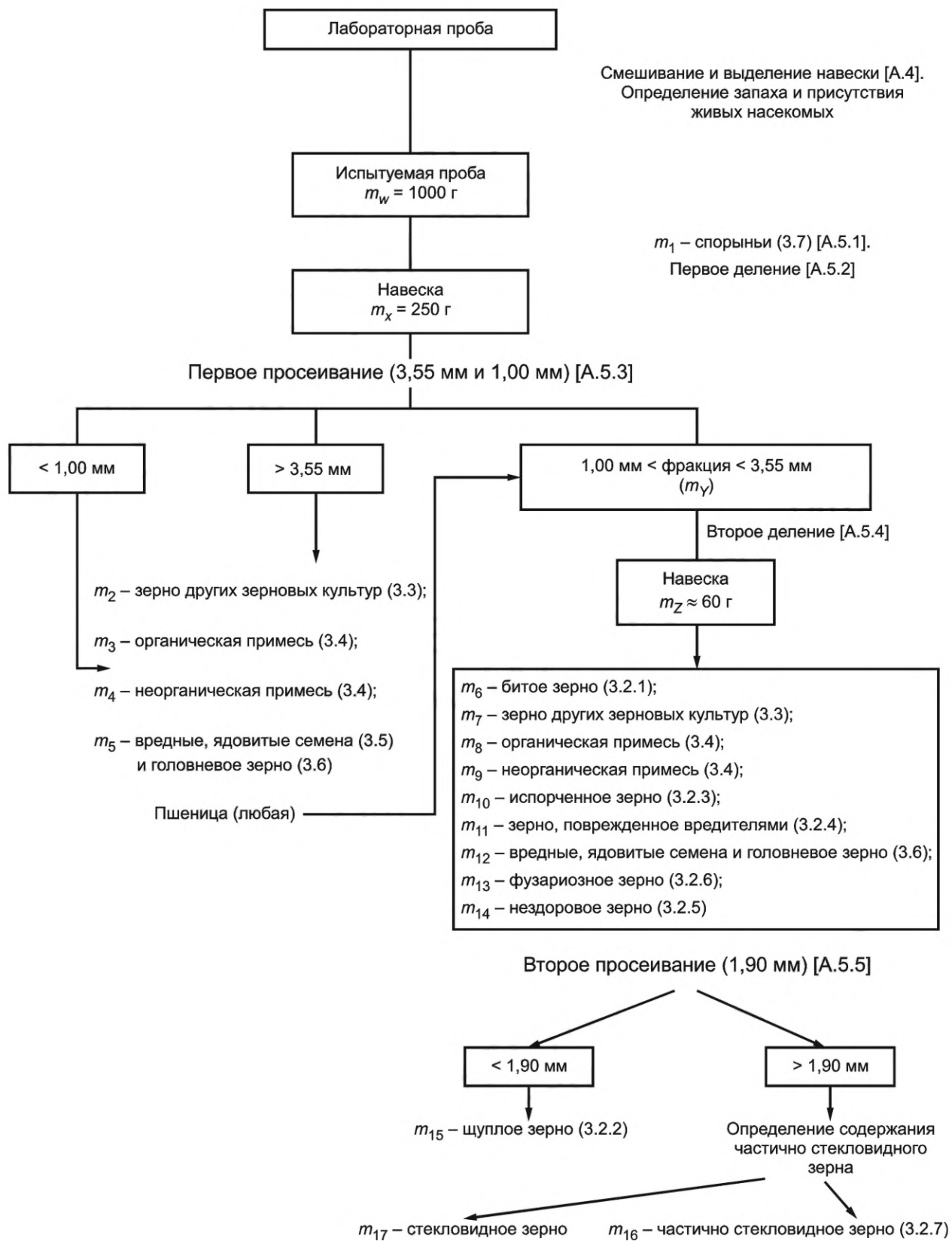
Рисунок А.1 — Схема проведения испытания
