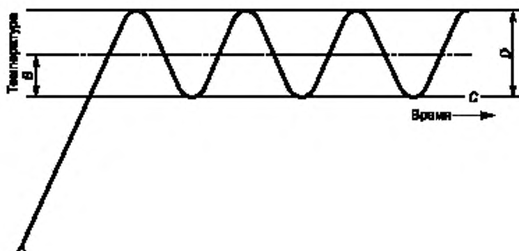
A — зарегистрированная температура; B — максимальное допустимое отклонение; C — минимальная регламентированная температура; D — область температуры стерилизации
