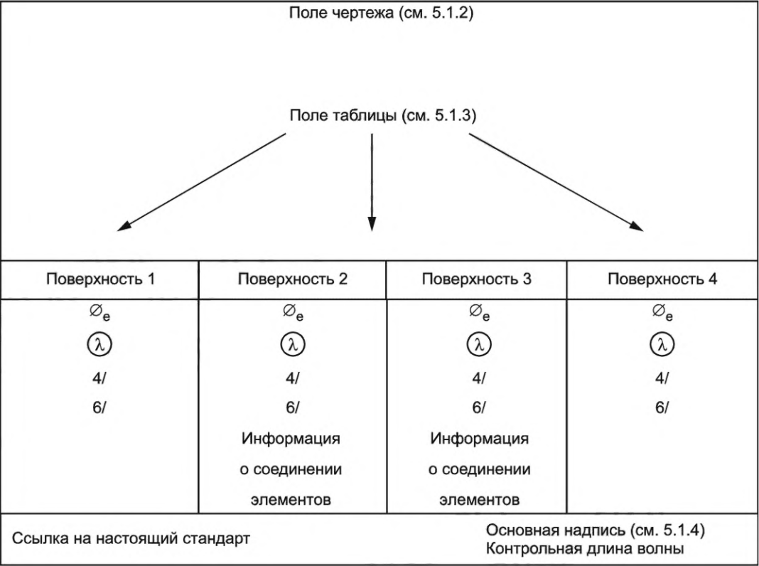
Рисунок 2 — Табличный формат оформления чертежа сборочной единицы
