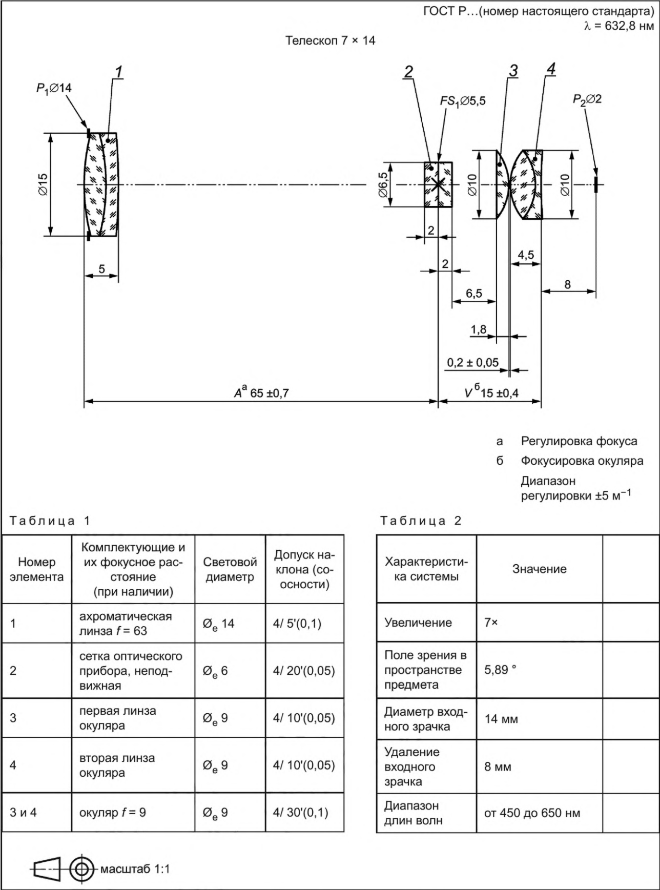
Рисунок 35 — Чертеж оптической системы
