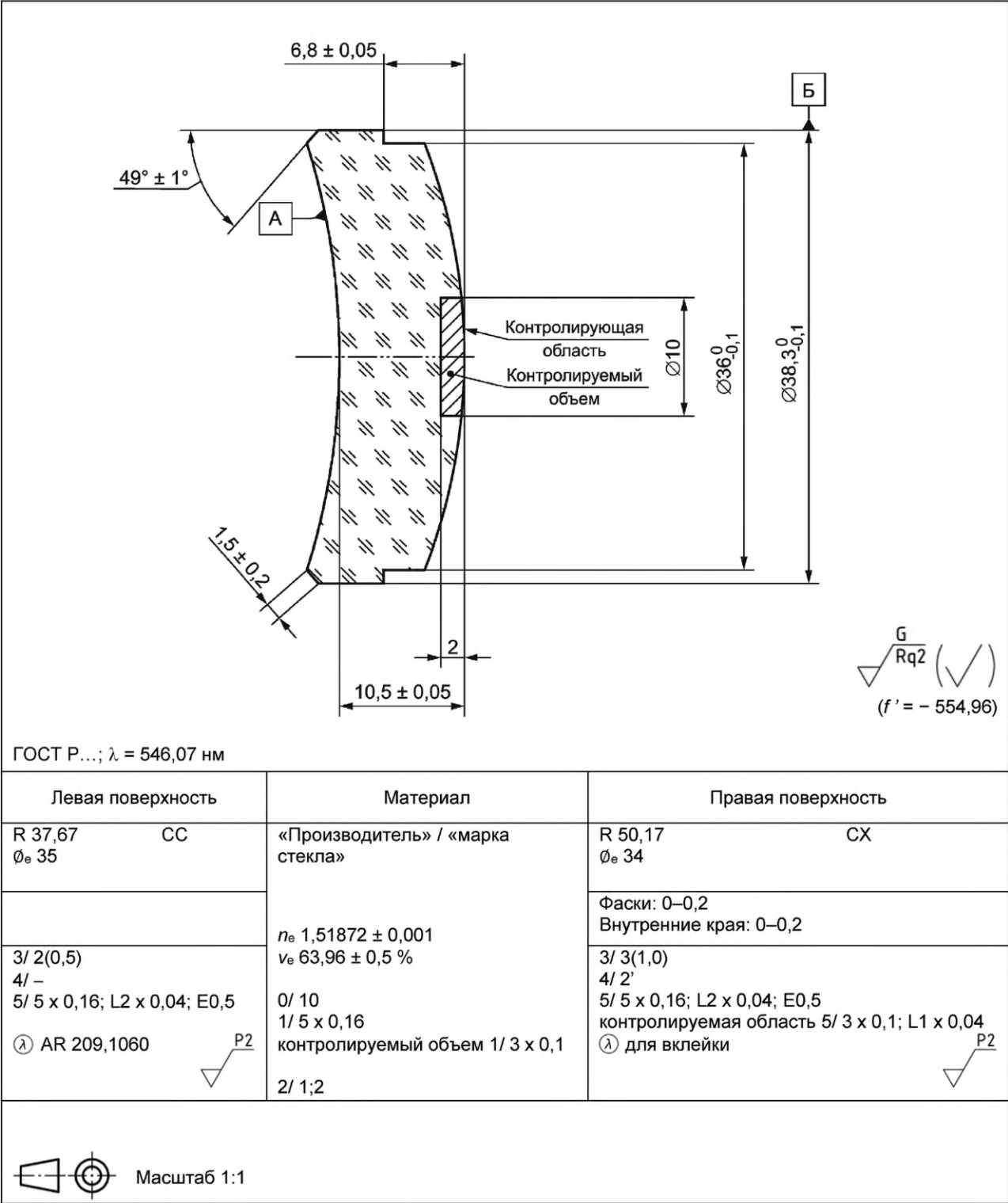
Рисунок А.2 — Чертеж линзы с указанием контролируемой области и контролируемого объема
