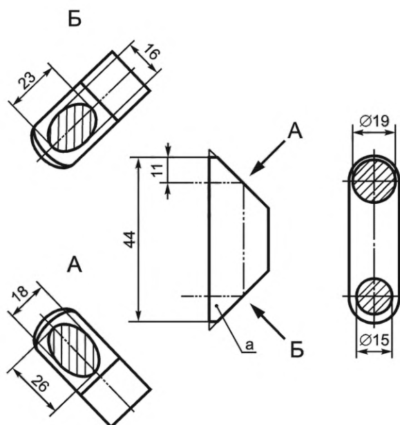
Рисунок 15 — Обозначение областей контроля призмы
