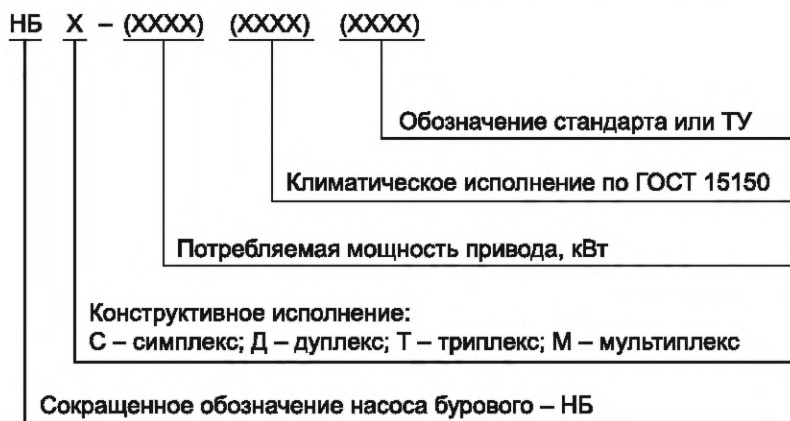
Рисунок 1 — Структура условного обозначения бурового насоса
