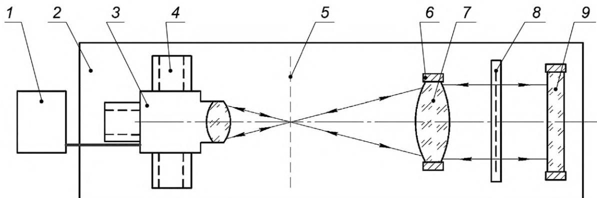
1 — регистрирующая аппаратура; 2 — единое амортизационное основание; 3 — интерферометр; 4 — двух- или трехкоординатное устройство; 5 — плоскость изображения испытуемого объектива; 6 — объективодержатель; 7 — испытуемый объектив; 8 — узел перемещения нити; 9 — плоское автоколлимационное зеркало
