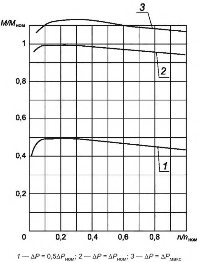
Рисунок Б.1 — Зависимость крутящего момента от частоты вращения
