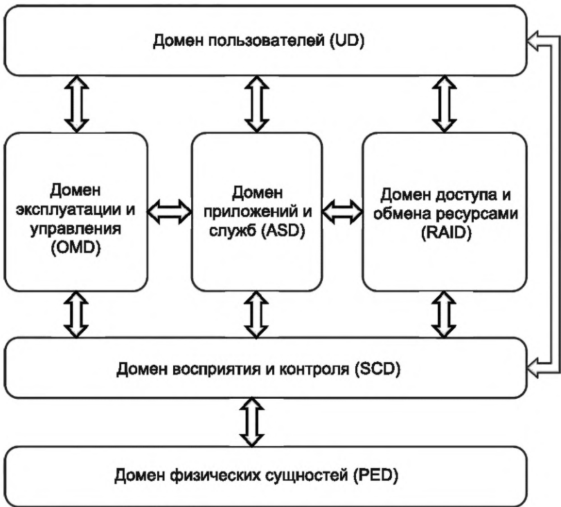
Рисунок 13 — Типовая модель на основе доменов
