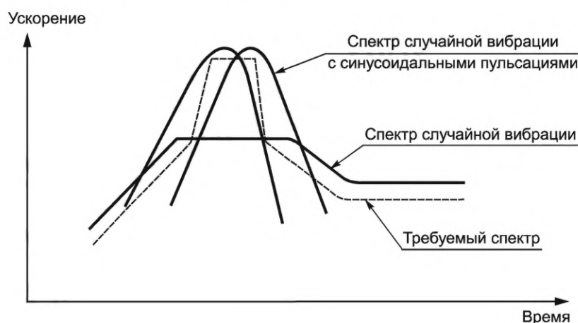
Рисунок 3 — Спектр случайной вибрации с наложенными синусоидальными пульсациями
