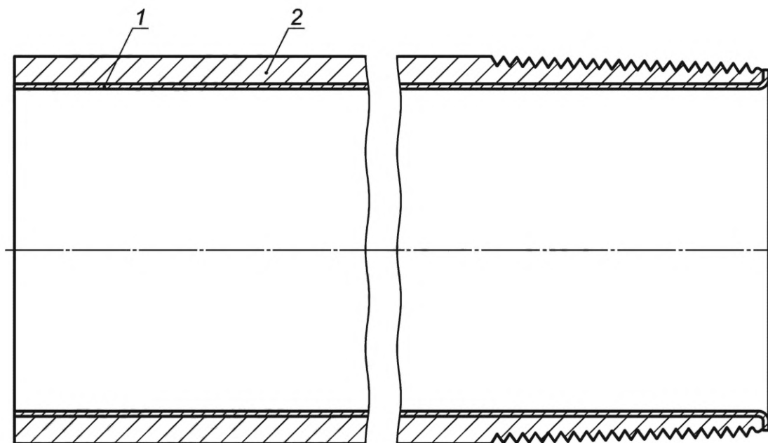
1 — лайнер; 2 — НКТ
