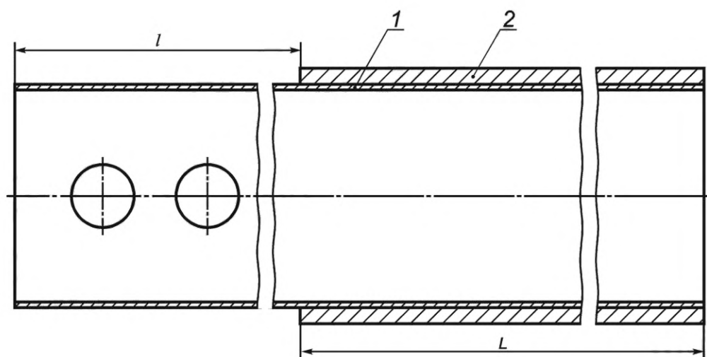
1 — лейнер; 2 — НКТ
