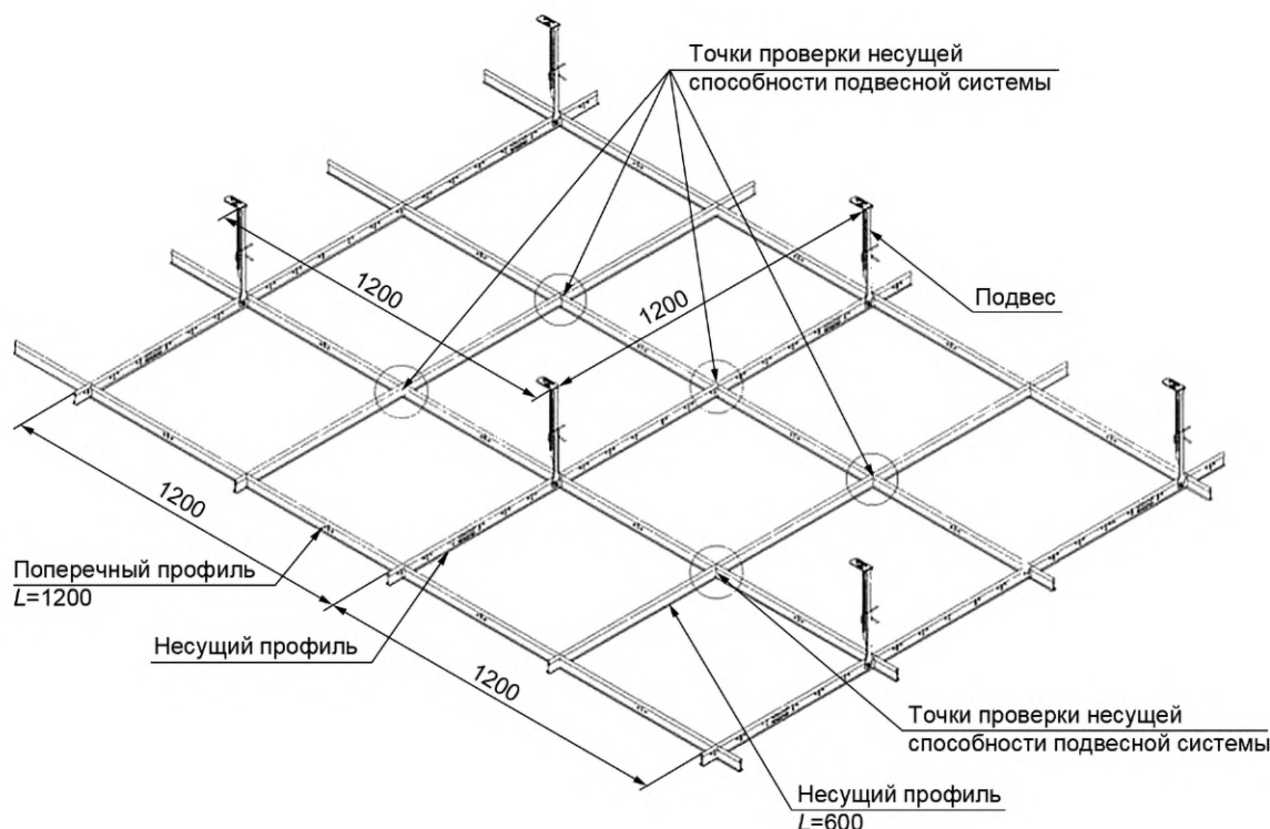
Рисунок А.1 — Схема монтажа подвесной системы для проведения испытаний на несущую способность
