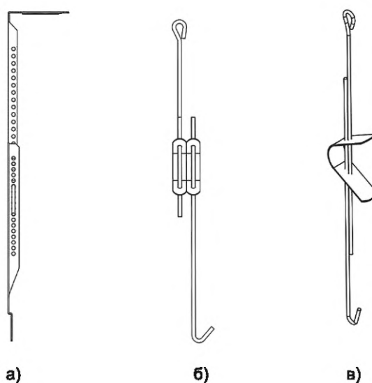
а) — жесткий регулируемый подвес; б), в) — проволочные регулируемые подвесы с зажимом из пружинной стали
