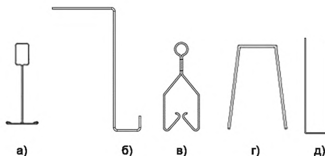
а) — несущий профиль для кассетного подвесного потолка; б) — несущий профиль для крупноформатных панелей скрытого типа крепления; в) — несущий профиль для панелей скрытого типа крепления; г) — несущий профиль для реечных потолков; д) — несущий П-профиль для решетчатого подвесного потолка
