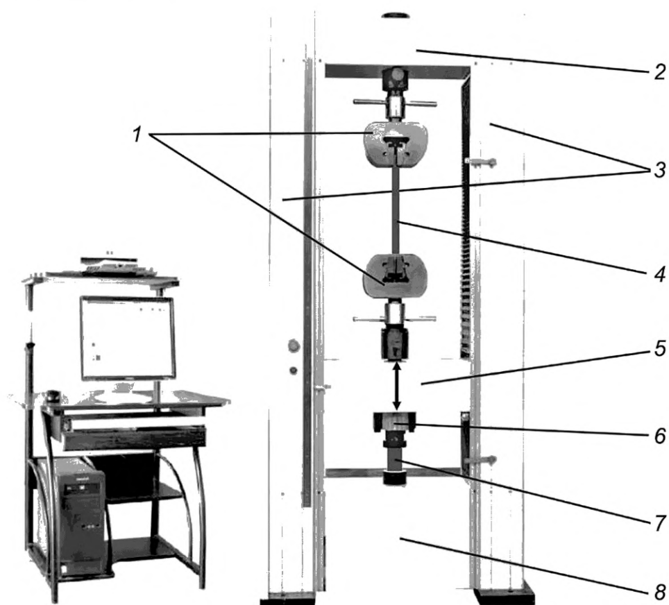
1 — захваты; 2 — силовая балка; 3 — колонны; 4 — образец № 1 (на растяжение); 5 — траверса; 6 — пресс; 7 — образец № 2 (на сжатие); 8 — основание
