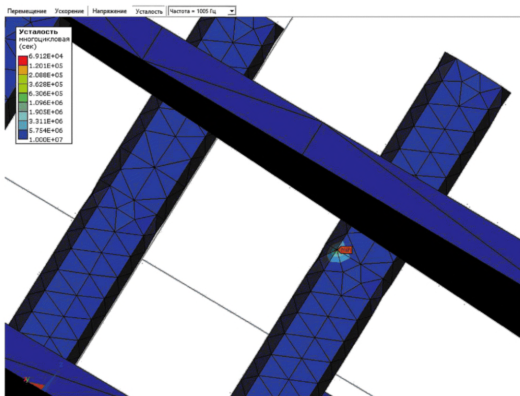
Рисунок А.9 — Время до усталостного разрушения во всех точках конструкции блока ЭА на резонансной частоте
