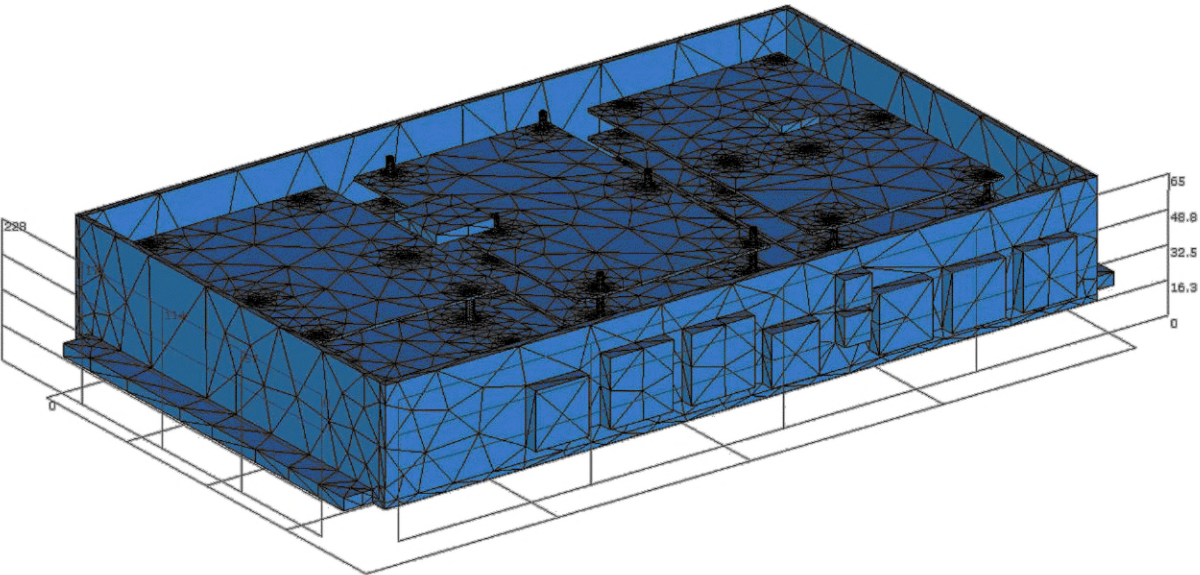
Рисунок А.5 — Автоматическое разбиение на конечные элементы
