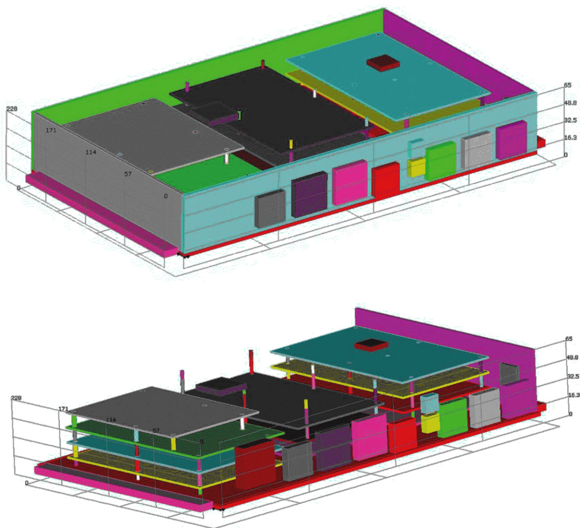
Рисунок А.4 — Конструкция блока ЭА, импортированная из CAD-системы в подсистему АСОНИКА-М-3D
