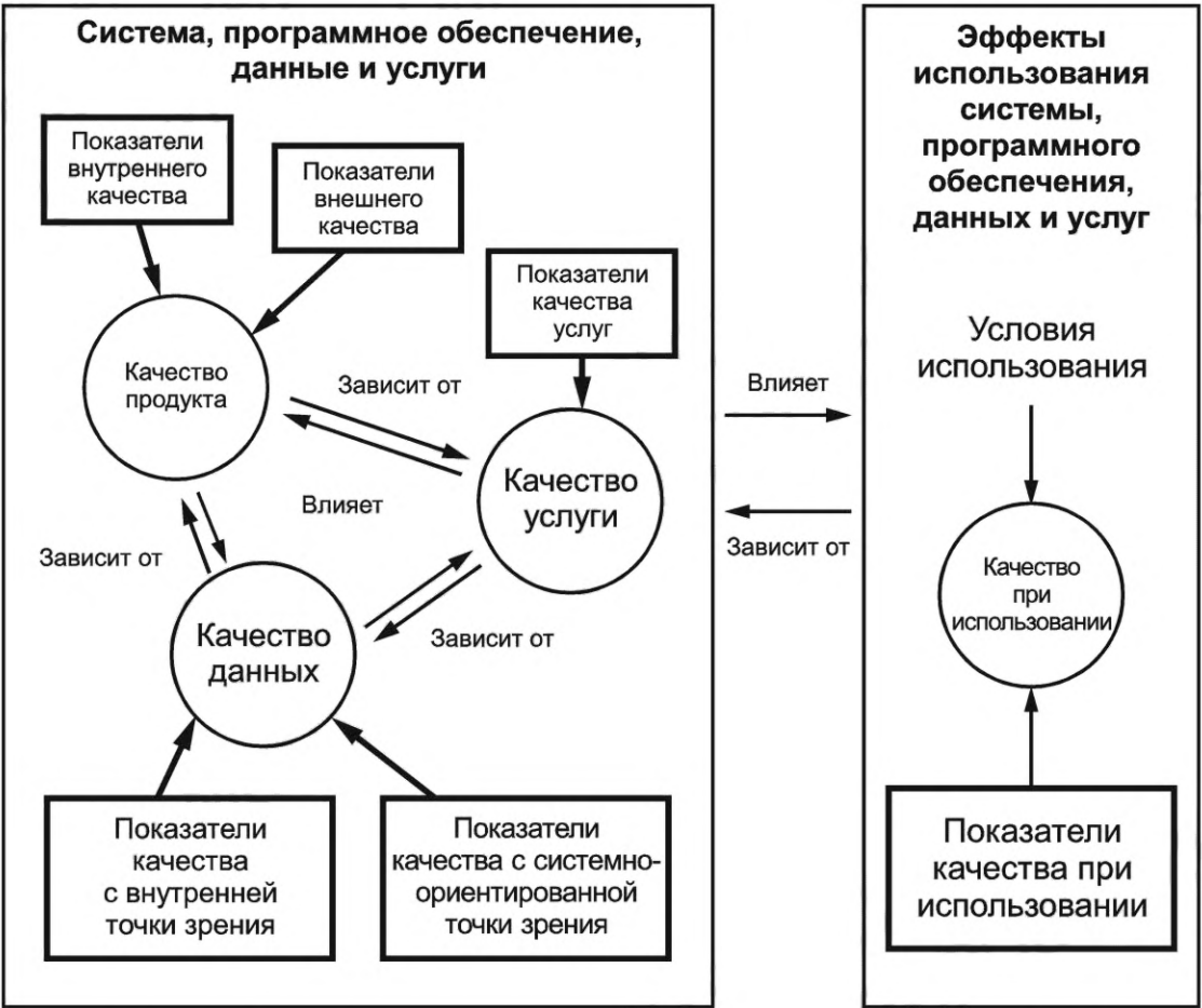
Рисунок 2 — Взаимосвязь между различными моделями качества из серии SQuaRE
