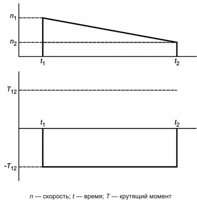
Рисунок 4 — Скорость вращения электродвигателя и тормозной момент при рекуперативном торможении
