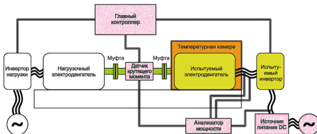
Рисунок 1 — Пример испытательной установки
