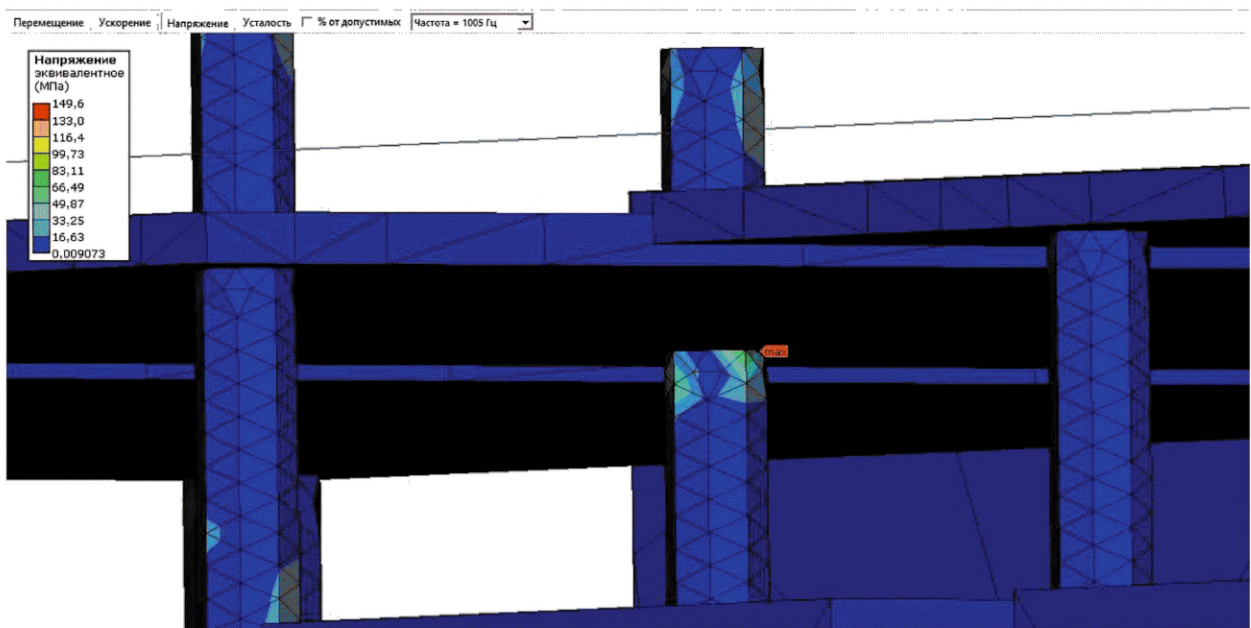
Рисунок А.8 — Эквивалентные механические напряжения во всех точках конструкции блока ЭА на резонансной частоте
