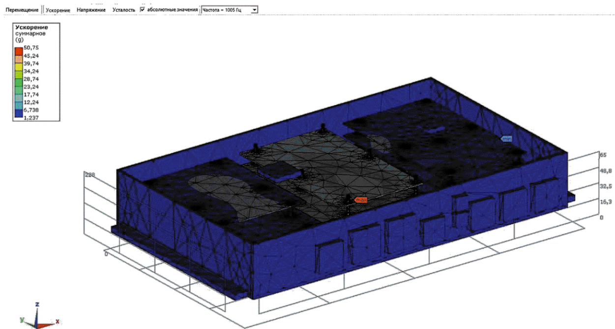
Рисунок А.7 — Суммарные ускорения во всех точках конструкции блока ЭА на резонансной частоте
