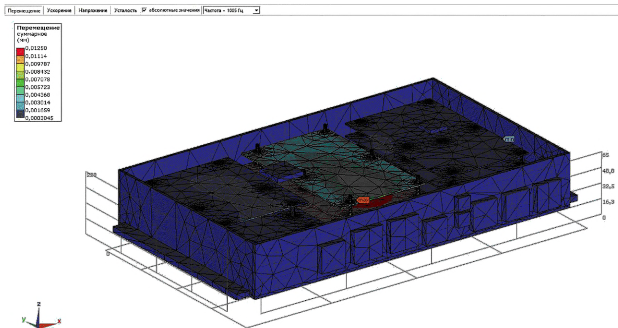
Рисунок А.6 — Суммарные перемещения во всех точках конструкции блока ЭА на резонансной частоте
