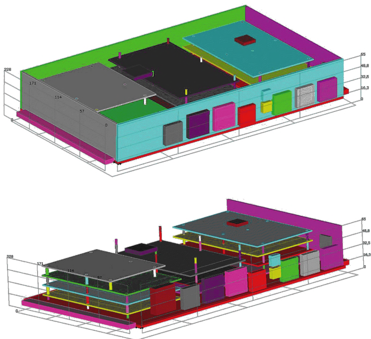
Рисунок А.1 — Конструкция блока ЭА, импортированная из CAD-системы в подсистему АСОНИКА-М-3D
