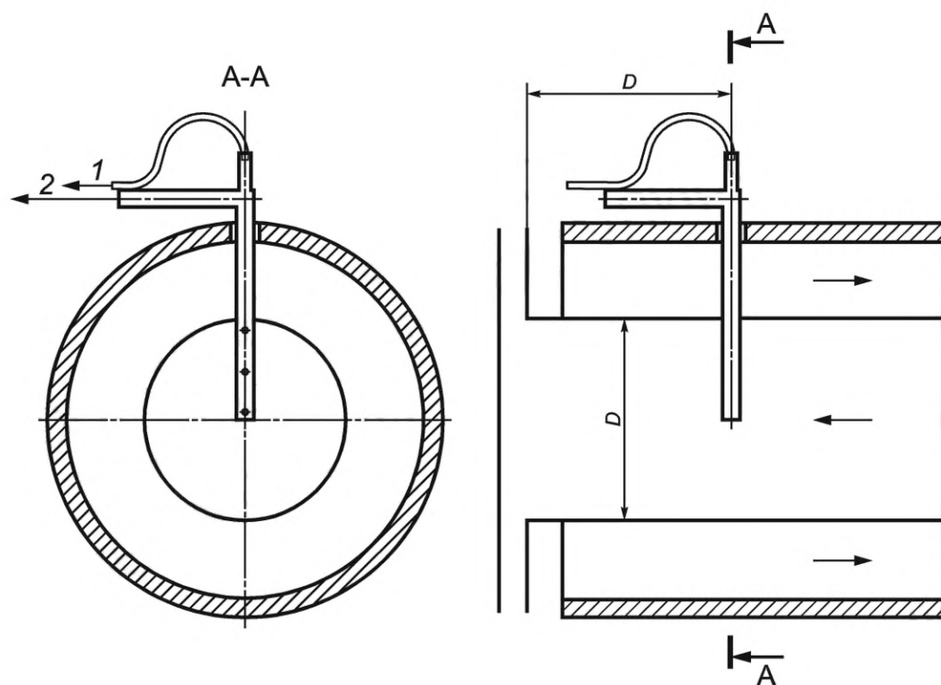
Рисунок К.5 — Расположение пробоотборника для аппаратов типов C_{12} и C_{13}
