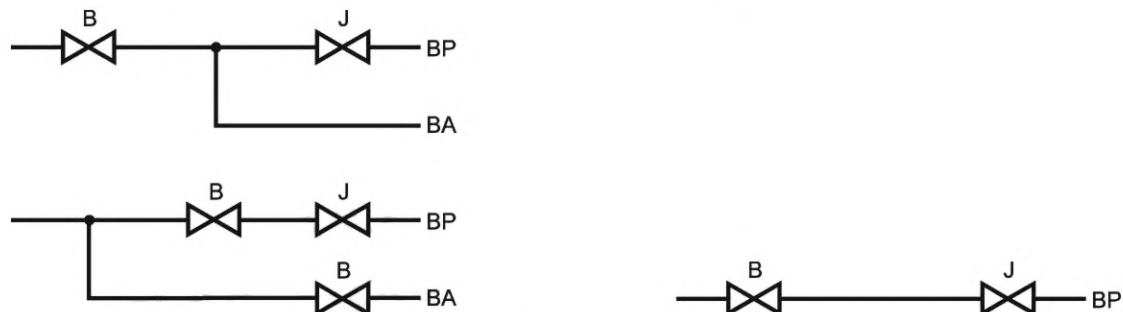
а) Аппарат с пилотной горелкой тепловой мощностью не более 1 кВт или 5 % от тепловой мощности основной горелки
