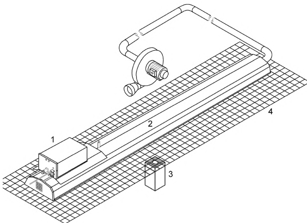
б) Обогреватель системы из непрерывных трубчатых излучающих обогревателей с несколькими горелками
