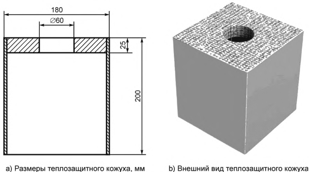
Рисунок 9 — Теплозащитный кожух
