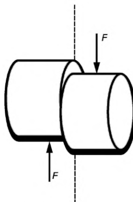
Рисунок 3 — Схема испытания
