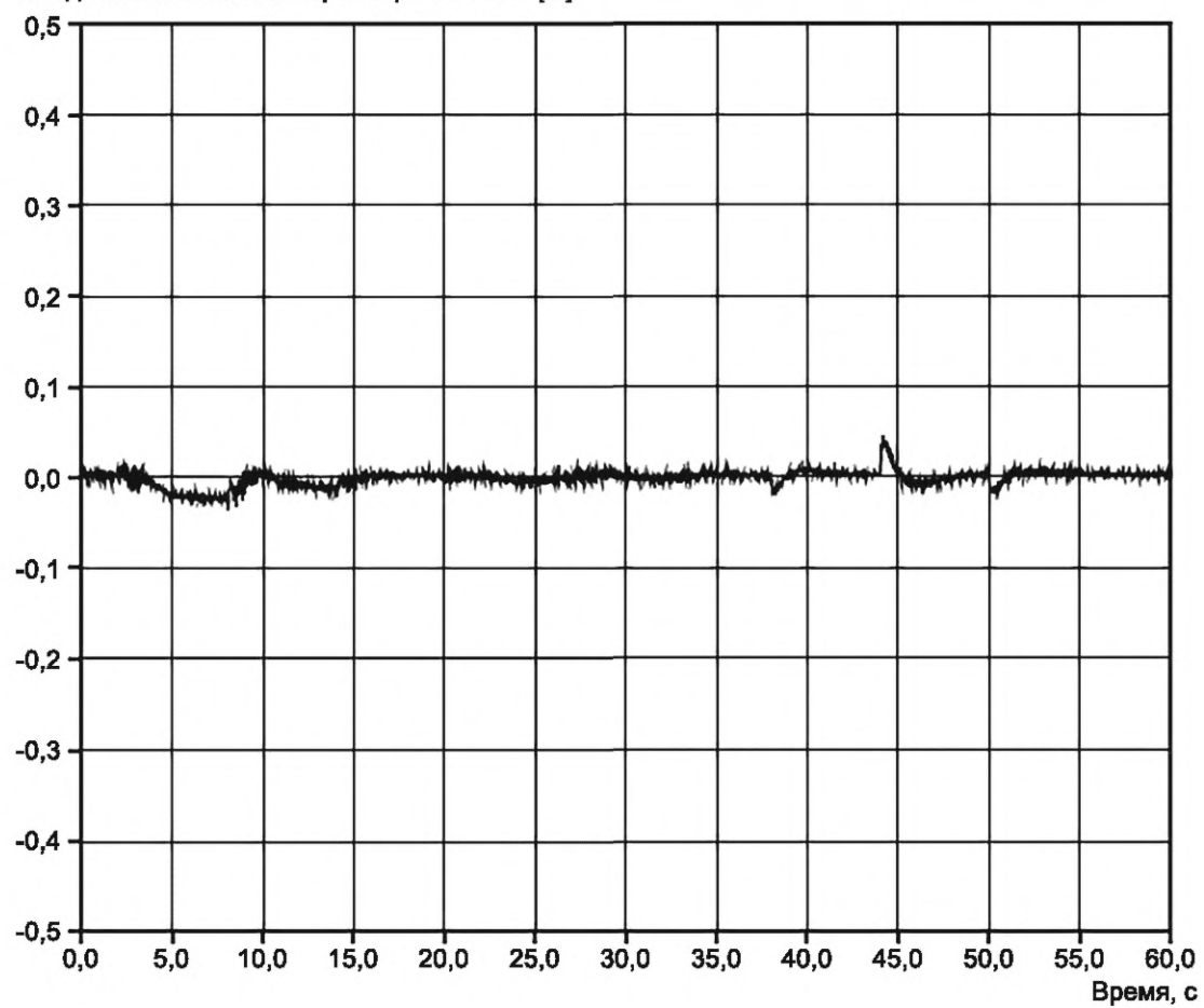
Рисунок 8 — Реакция на входные сигналы линейного ускорения по оси Z
