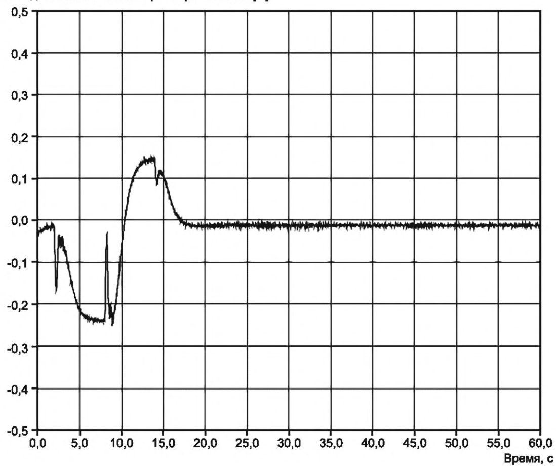
Рисунок 6 — Реакция на входные сигналы линейного ускорения по оси X
