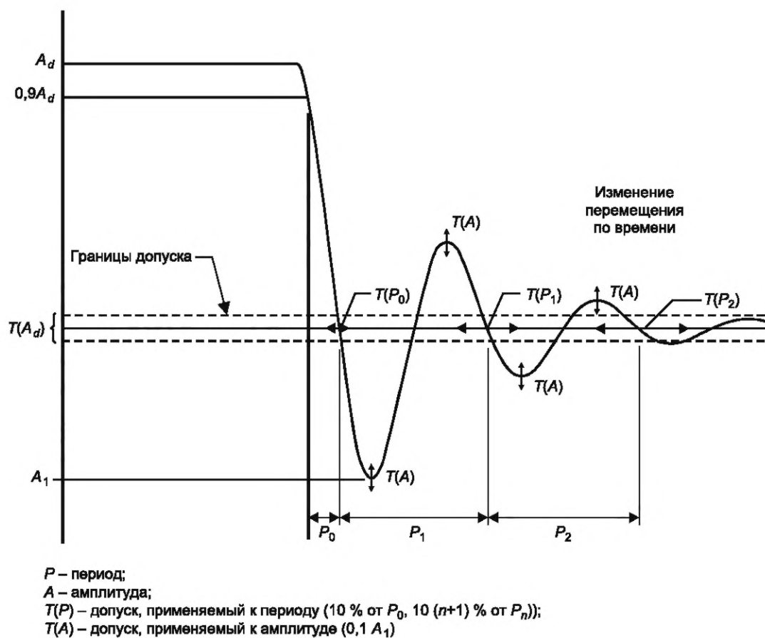
Рисунок 1 — Характеристика переходного процесса с недостаточным демпфированием
