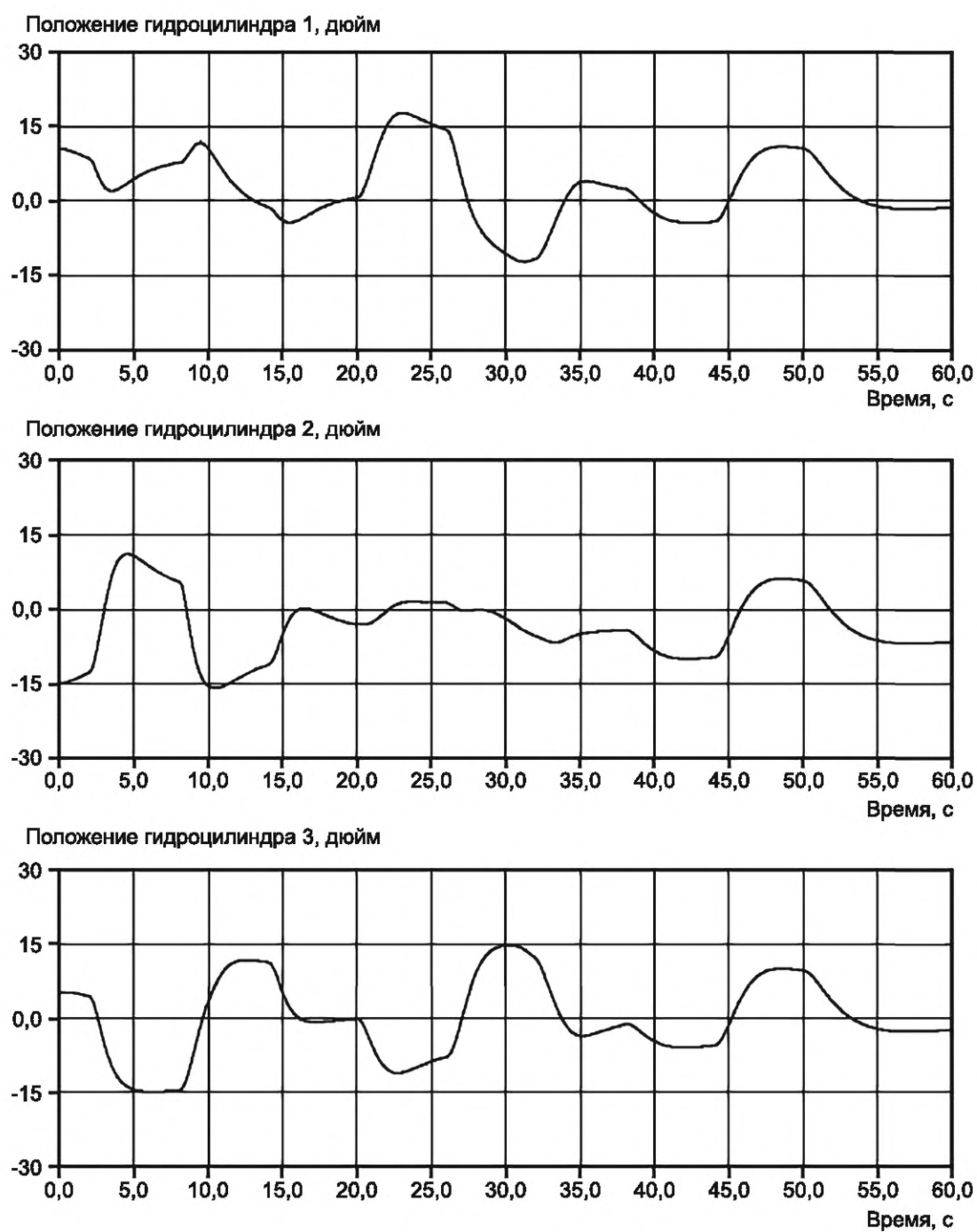
Рисунок 9 — Положение гидроцилиндров 1—3
