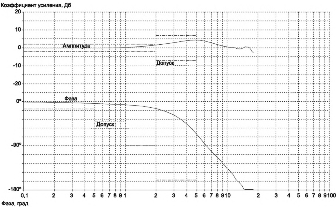
Рисунок 3 — Диаграмма Боде
