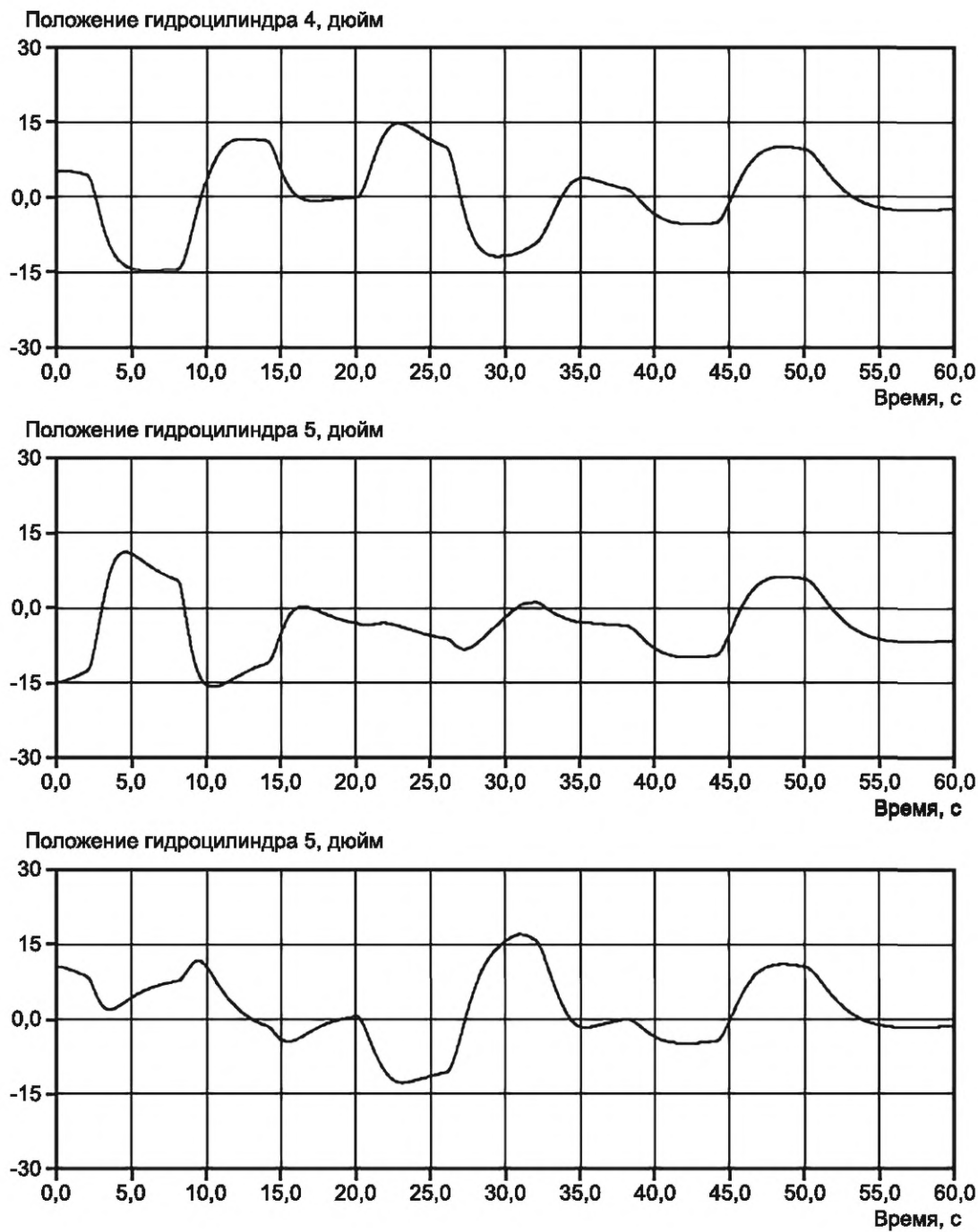
Рисунок 10 — Положение гидроцилиндров 4—6
