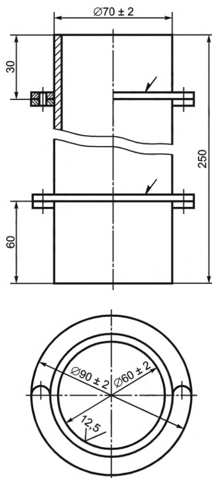
Рисунок 6 — Разъемный кожух
