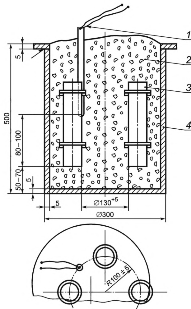
1 — хромель-алюмелевая термопара в чехле; 2 — пересыпочный кокс; 3 — кожух с массой; 4 — контейнер
