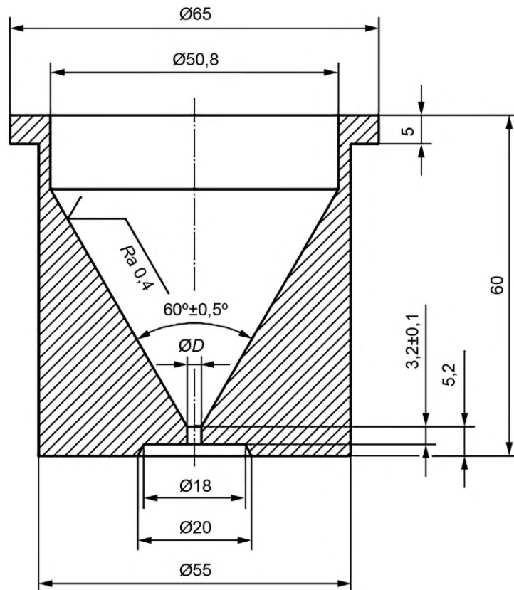
Рисунок 1 — Воронка Холла
