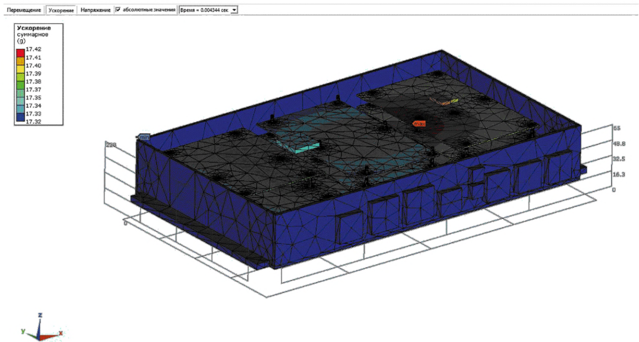
Рисунок А.7 — Суммарные ускорения во всех точках конструкции блока ЭА при воздействии одиночного механического удара в заданный момент времени
