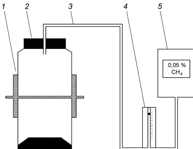
1 — сдвигательное устройство; 2 — камера десорбции; 3 — шланг; 4 — устройство учета газа (расходомер); 5 — газоанализатор
