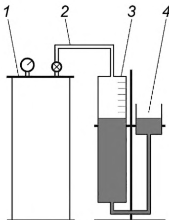
1 — камера десорбции; 2 — шланг; 3 — бюретка; 4 — чаша подпитки
