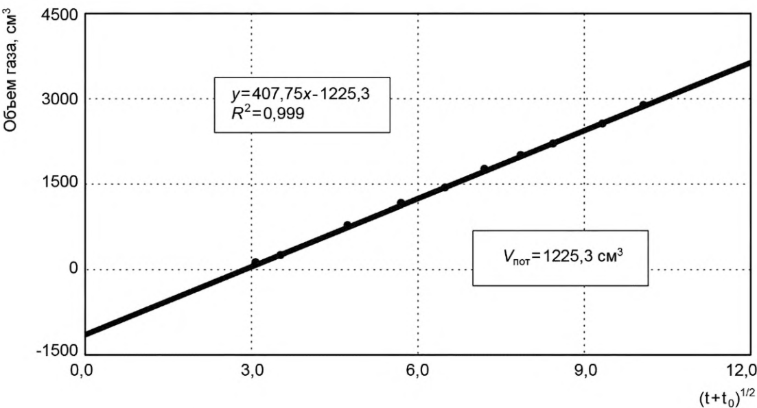
Рисунок С.1 — График расчета объема потерь газа
