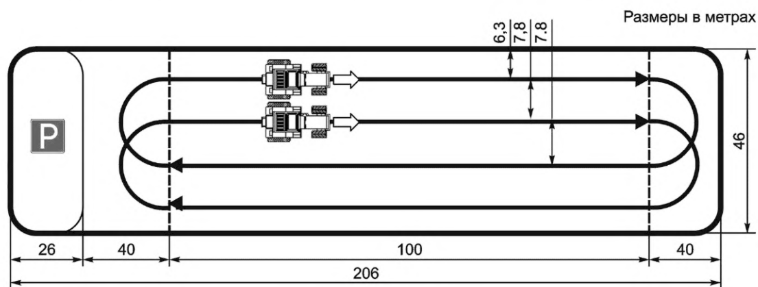
Рисунок А.1 — Минимальные размеры площадки для тестирования при движении в параллельном потоке
