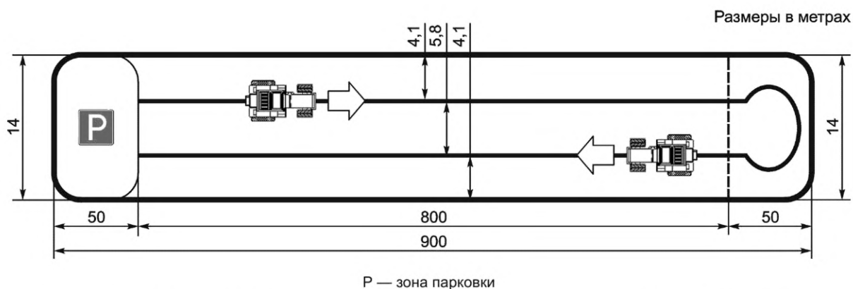
Рисунок А.3 — Минимальные размеры площадки для тестирования при прямолинейном движении
