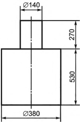
Рисунок В.1 — Испытательный объект, имитирующий сидящего человека
