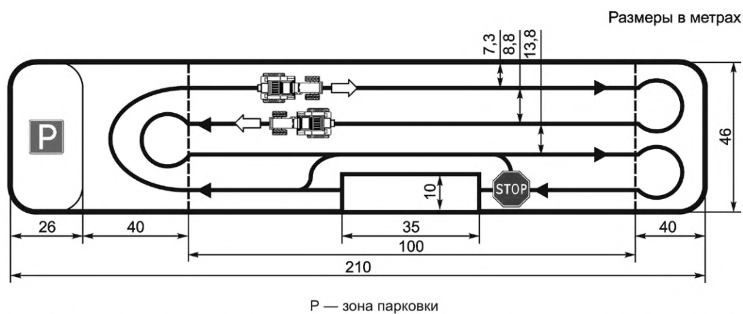
Рисунок А.2 — Минимальные размеры площадки для тестирования при движении во встречном потоке
