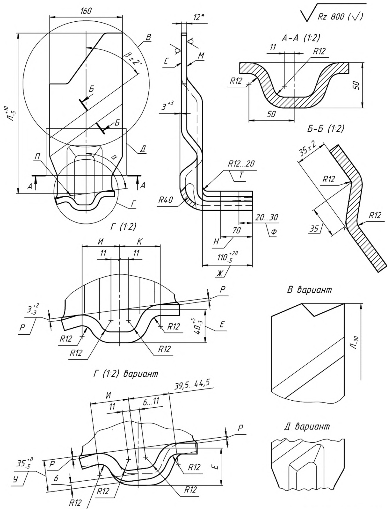
Рисунок 1 — Упоры крышек люков, тип 1
