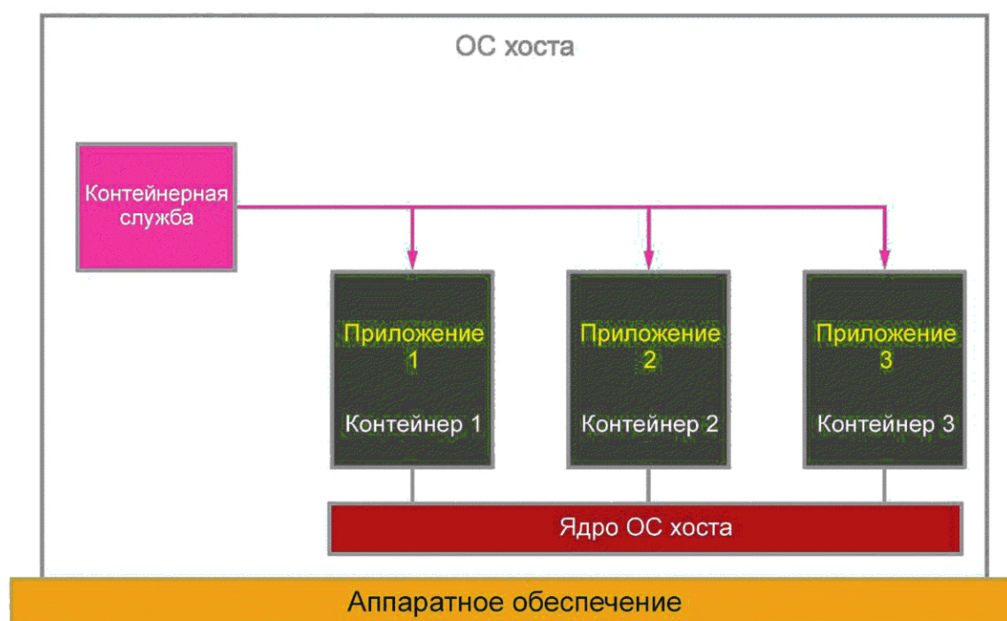
Рисунок 3 — Виртуализация контейнеров
